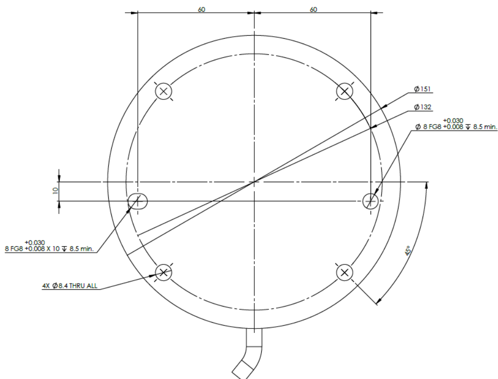
1.1: Vedea de jos bazei robotului
